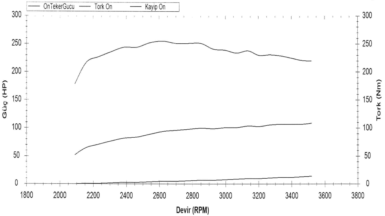
Dyno Testi Grafiği
